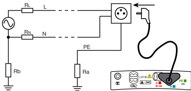
Caso de una instalación TT
